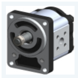
Насос GP2K16R-F281C-F
